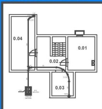
PÓDORYS VNÚTORNEJ KANALIZÁCIE
